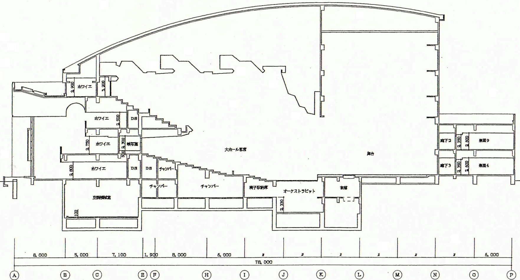
b-b断面図 1/200
